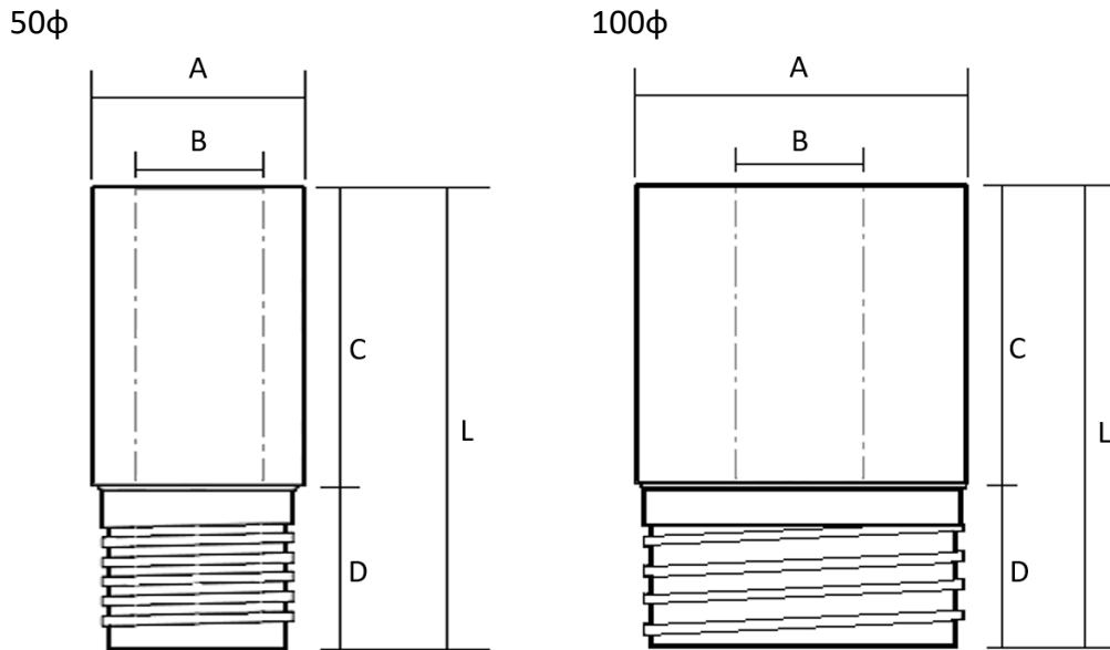
50φ用 吊り下げヘッド 寸法表
