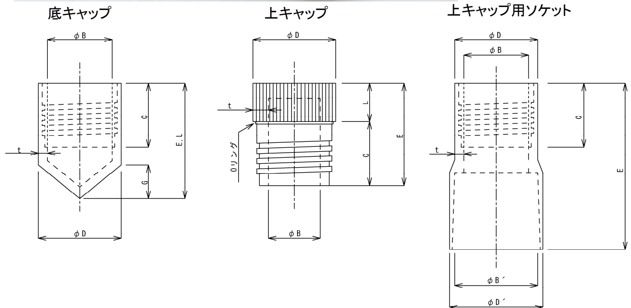
25φ用底キャップ および 上キャップ寸法表
